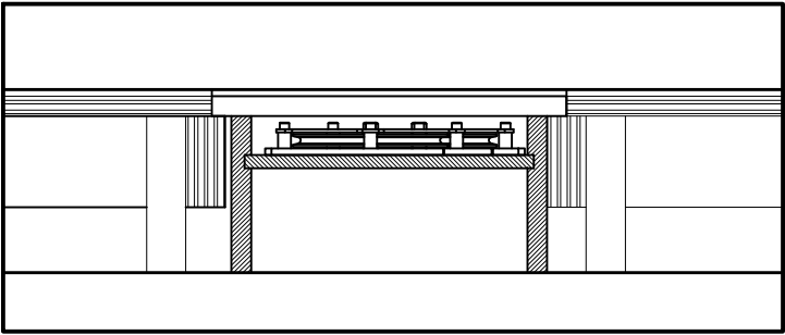
Detail B-B' Scale: 1 \frac{1}{2}" = 1'-0"
