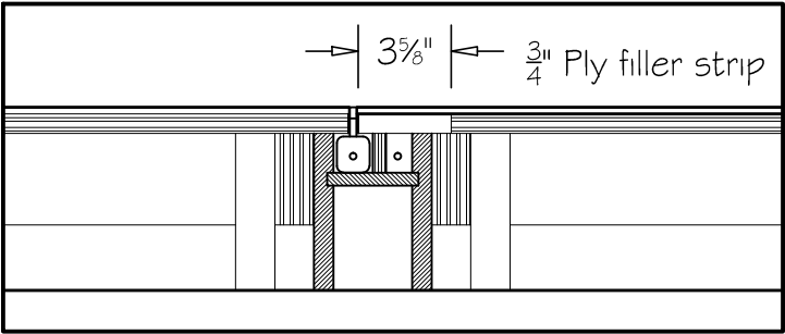
Detail A-A' Scale: 1 \frac{1}{2}" = 1'-0"
